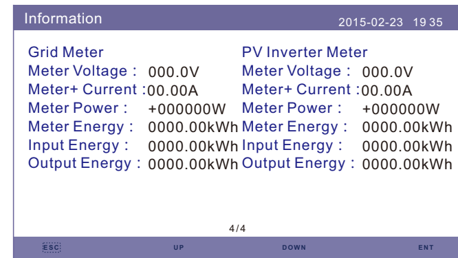
Abbildung 6.8 Informationsseite 4
