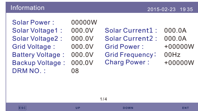
Abbildung 6.5 Informationsseite 1
