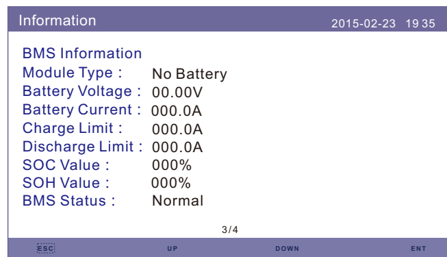
Abbildung 6.7 Informationsseite 3
