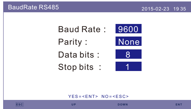
Abbildung 6.52 BaudRate RS485
