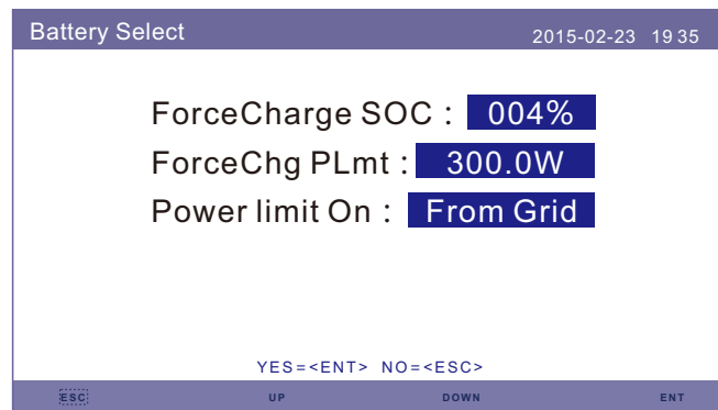
Abbildung 6.35 Zwangsladung SOC
