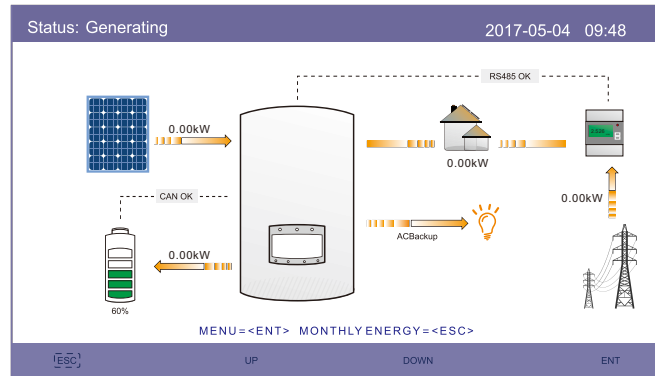
Abbildung 6.3 Hauptseite
